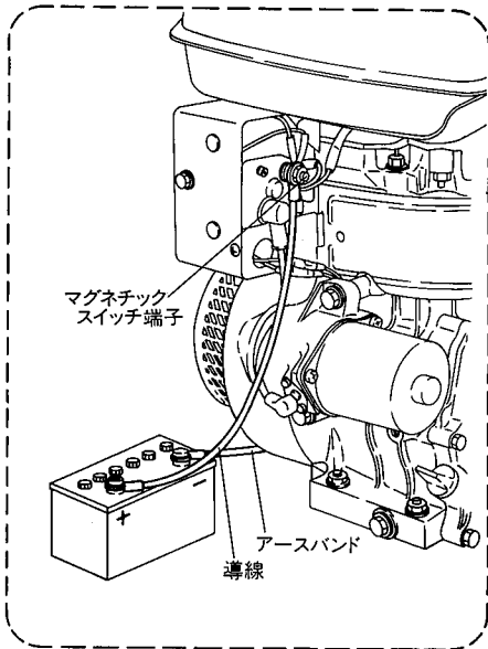
【配線図】
