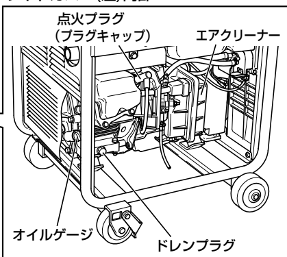
サイドカバー(左)内部
