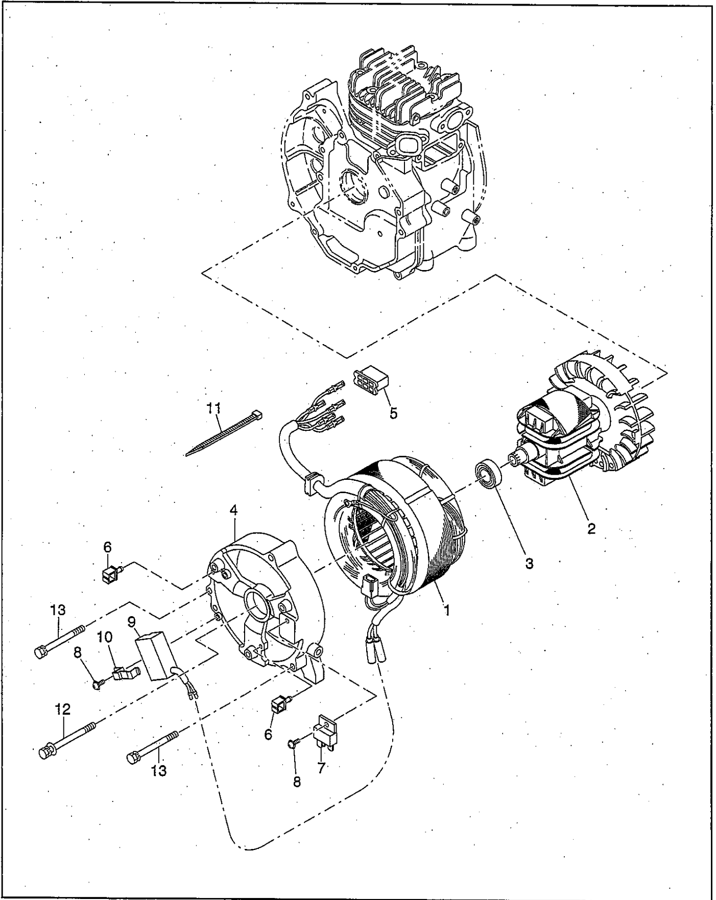
FIG.1 GENERATOR
