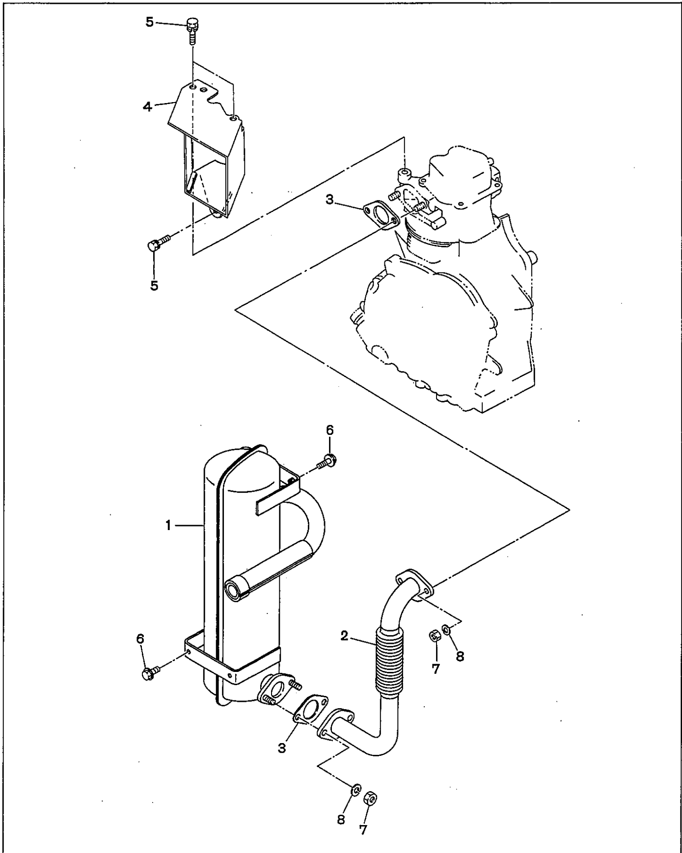
FIG. 6 MUFFLER
